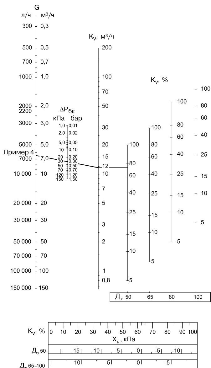
Диаграмма для выбора диаметра и условий регулирования клапанов ASV-PV D_y = 50-100 \text{ мм}
