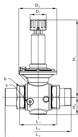
Размеры клапанов ASV-PV D v = 50 мм
