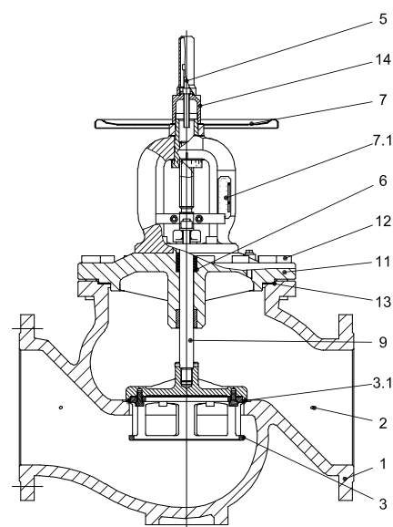
D_y = 65 мм
