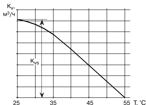
Характеристика регулирования клапана MTCV (базовая версия)
