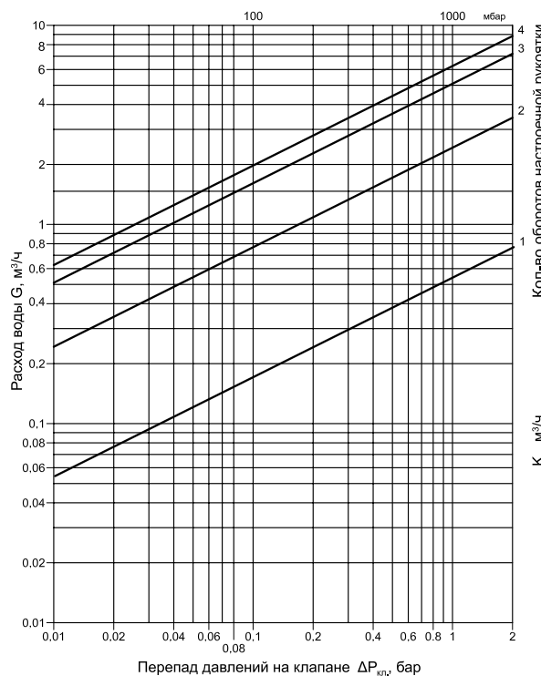
Диаграмма для настройки клапана MSV-F2 D_y = 20 мм
