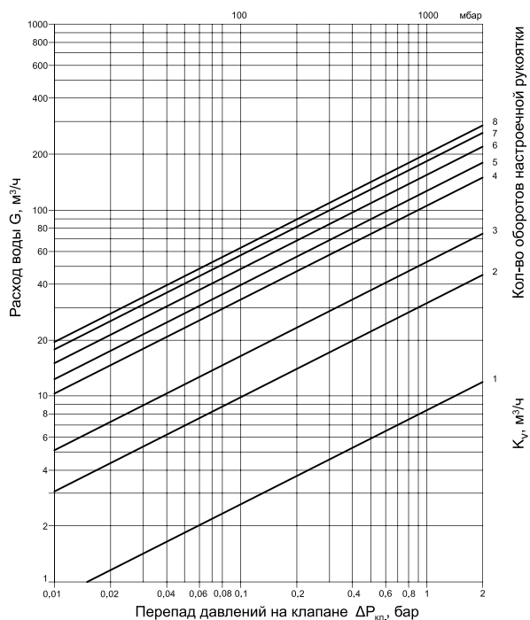
Диаграмма для настройки клапана MSV-F2 D_y = 100 мм
