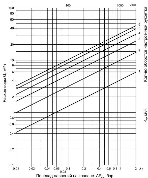
Диаграмма для настройки клапана MSV-F2 D_y = 40 мм
