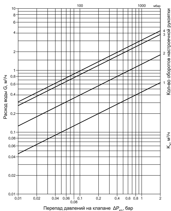
Диаграмма для настройки клапана MSV-F2 D_y = 15 мм
