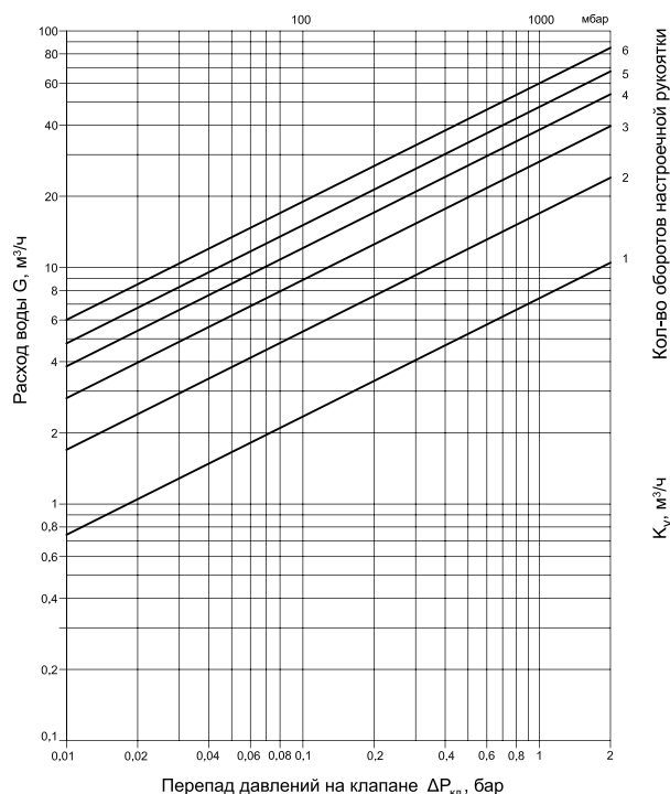
Диаграмма для настройки клапана MSV-F2 D_y = 50 мм
