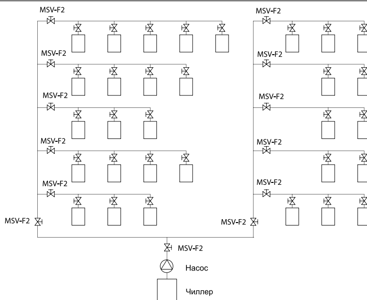
Пример применения клапана MSV-F2
