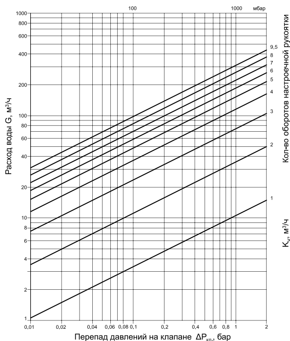
Диаграмма для настройки клапана MSV-F2 D_y = 125 мм
