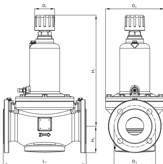
Размеры клапанов ASV-PV D v = 50 мм
