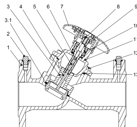
D_y = 65 мм
